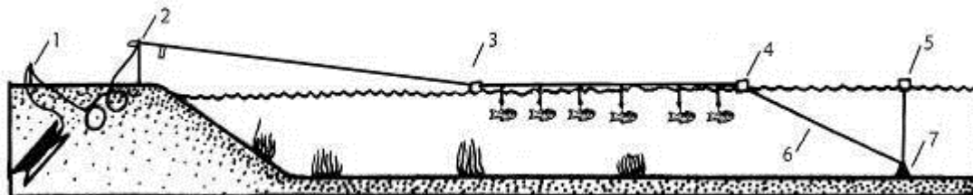
Рис. 5. Щучья резинка: 1 — кольшечек, надежно вбитый в берег; 2 — прут, в расщепе которого зажата основная леска; 3, 4 — поплавки; 5 — буйек (иногда не применяется); 6 — резиновый амортизатор; 7 — груз.
