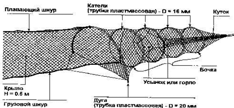
Рис. 49. Устройство современной сети (для удобства изображено лишь одно крыло).
